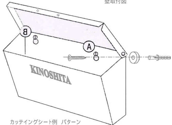
壁取付図
